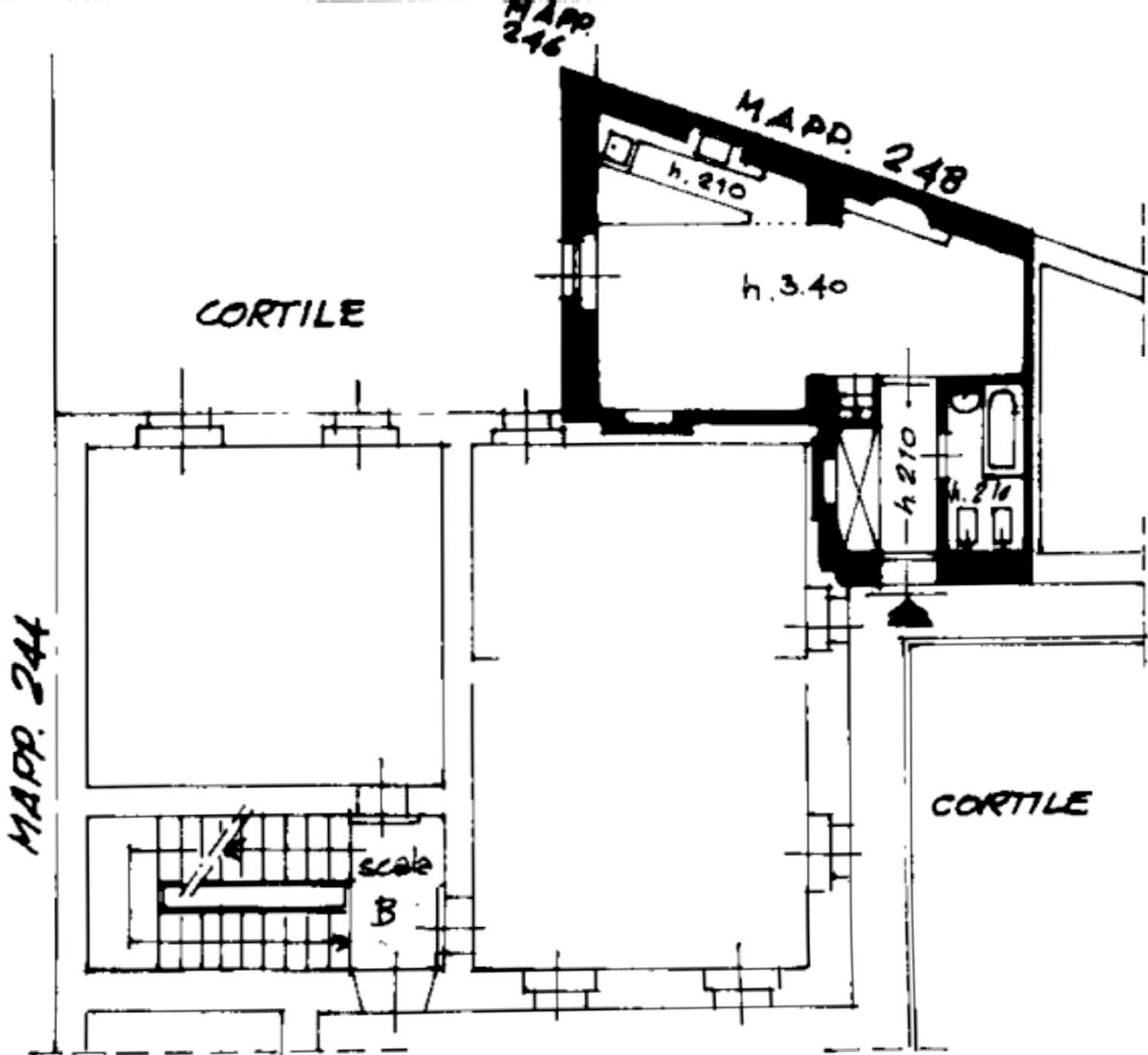
PIANO SECONDO
